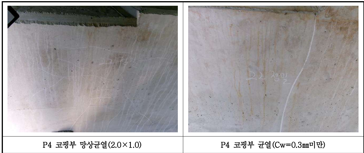
【사진 34.3.11】 교각 손상현황
