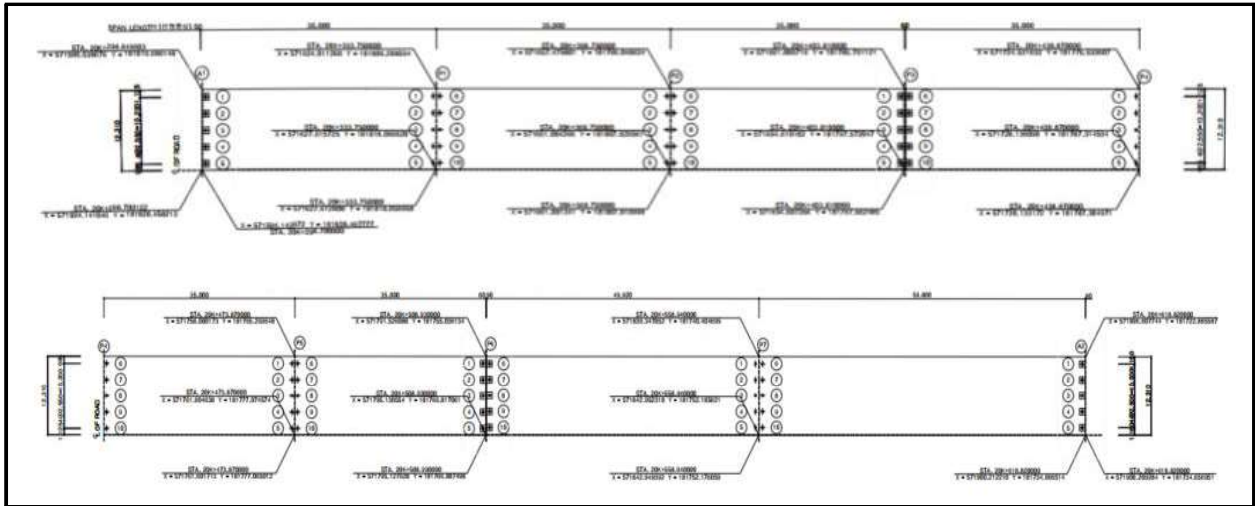
【그림 34.3.1】 교량받침 배치도
