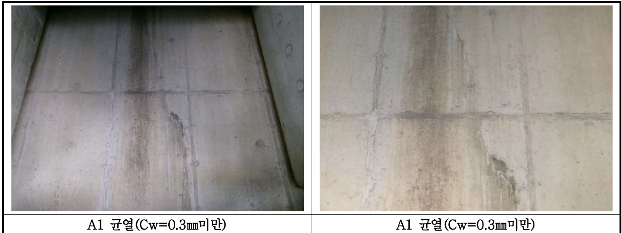
【사진 34.3.9】 교대 손상현황
