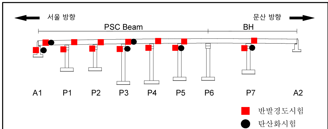
【그림 34.4.1】 콘크리트 내구성조사 위치도
