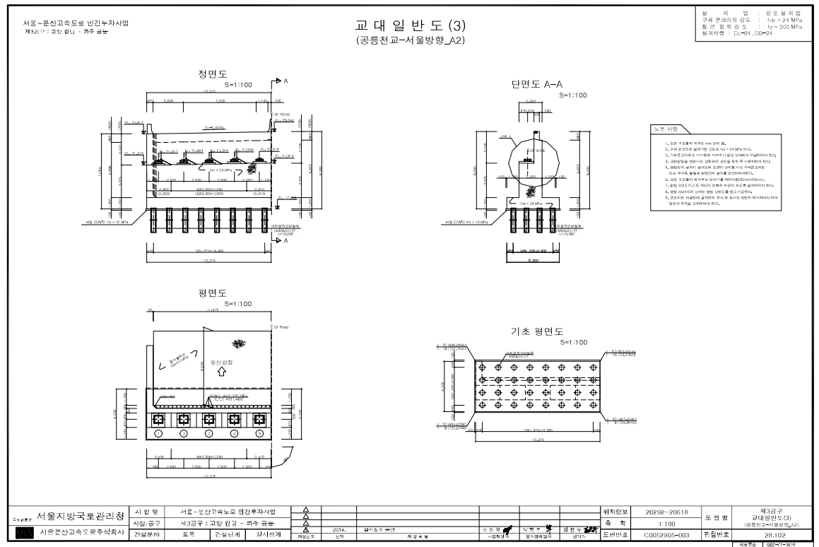
【그림 34.1.6】 교대 일반도
